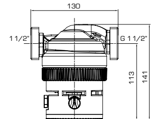
Laing Ecocirc® auto 25-130 G
