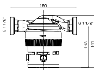
Laing Ecocirc® auto 25-180 G
