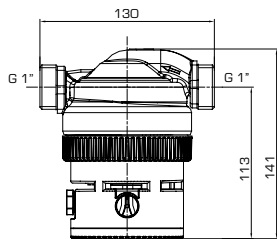
Laing Ecocirc® auto 15-130 G
